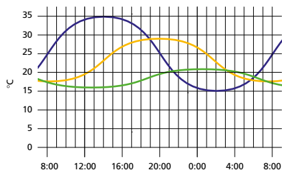
Průběh teploty na střeše při rozdílné izolaci
